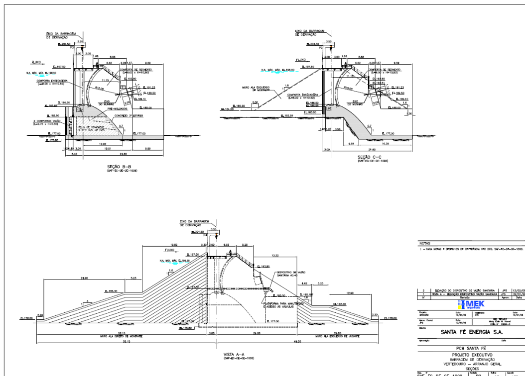
Figura 5 – Sistema extravasor
