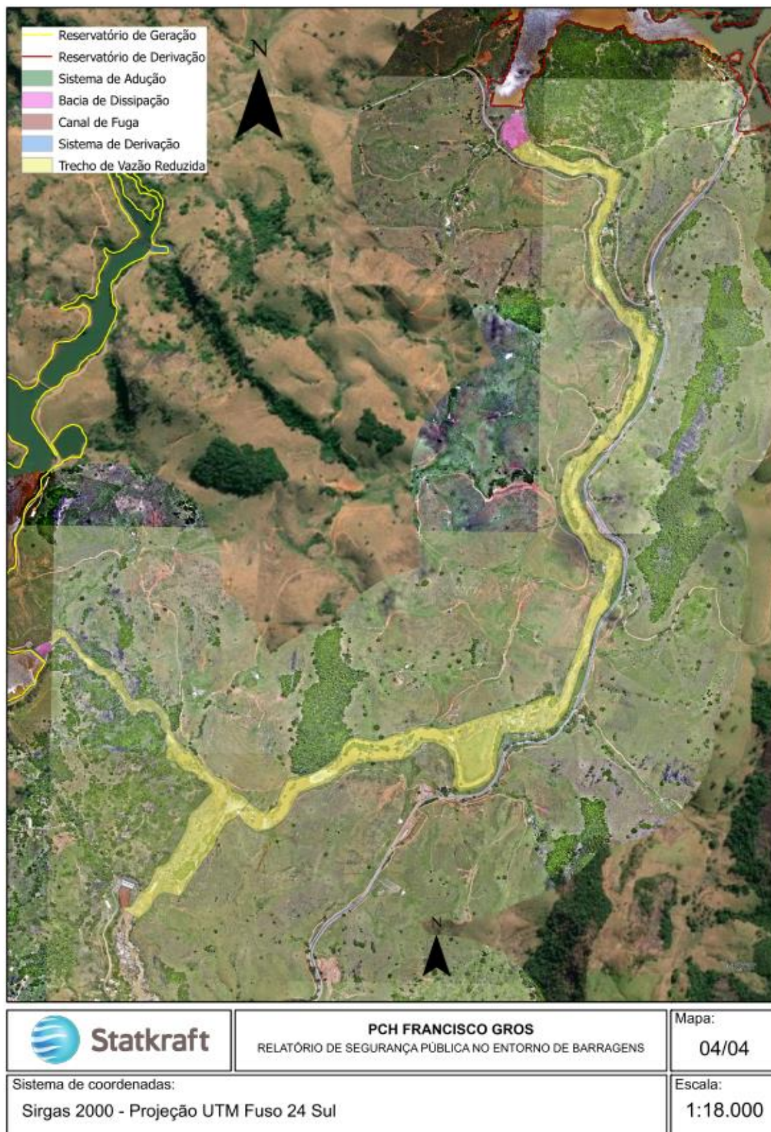
Figura 27 – Delimitação do trecho de vazão reduzida
