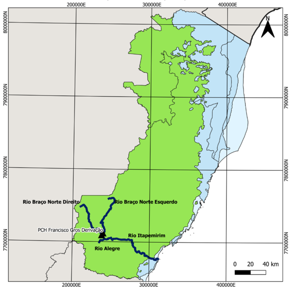
Figura 30 – Hidrogeologia
