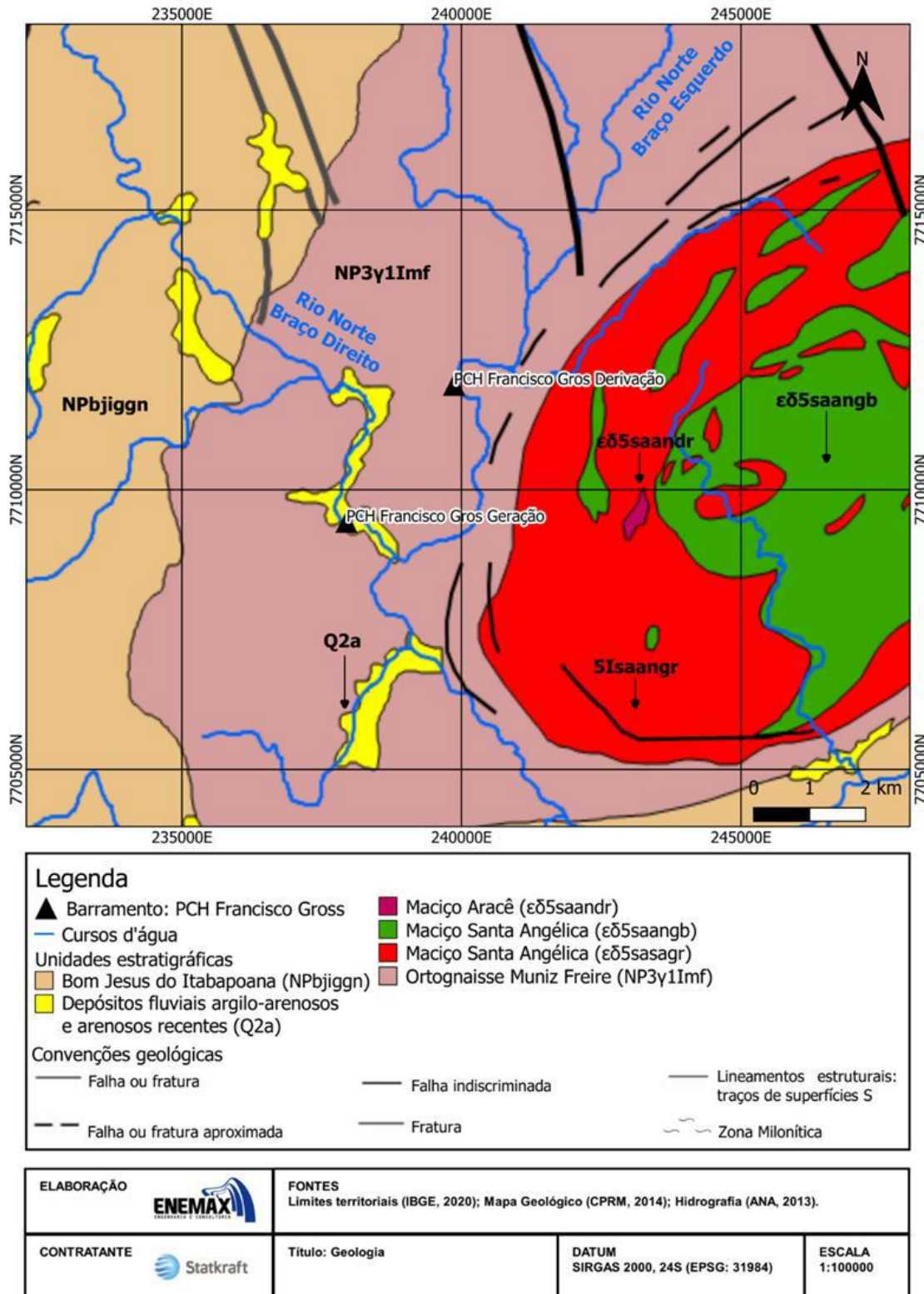
Figura 29 – Geologia regional
