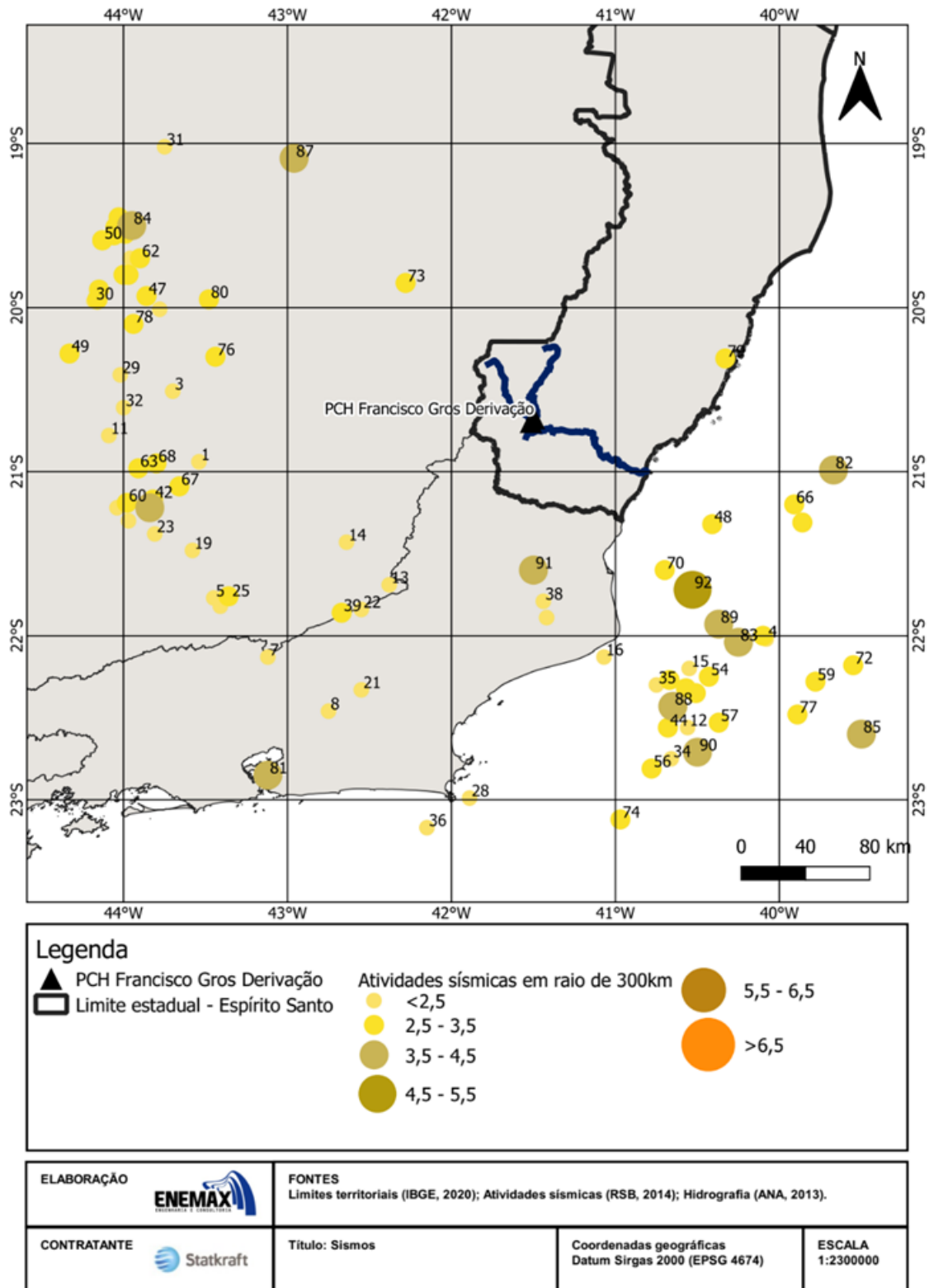
Figura 31 – Sismos
