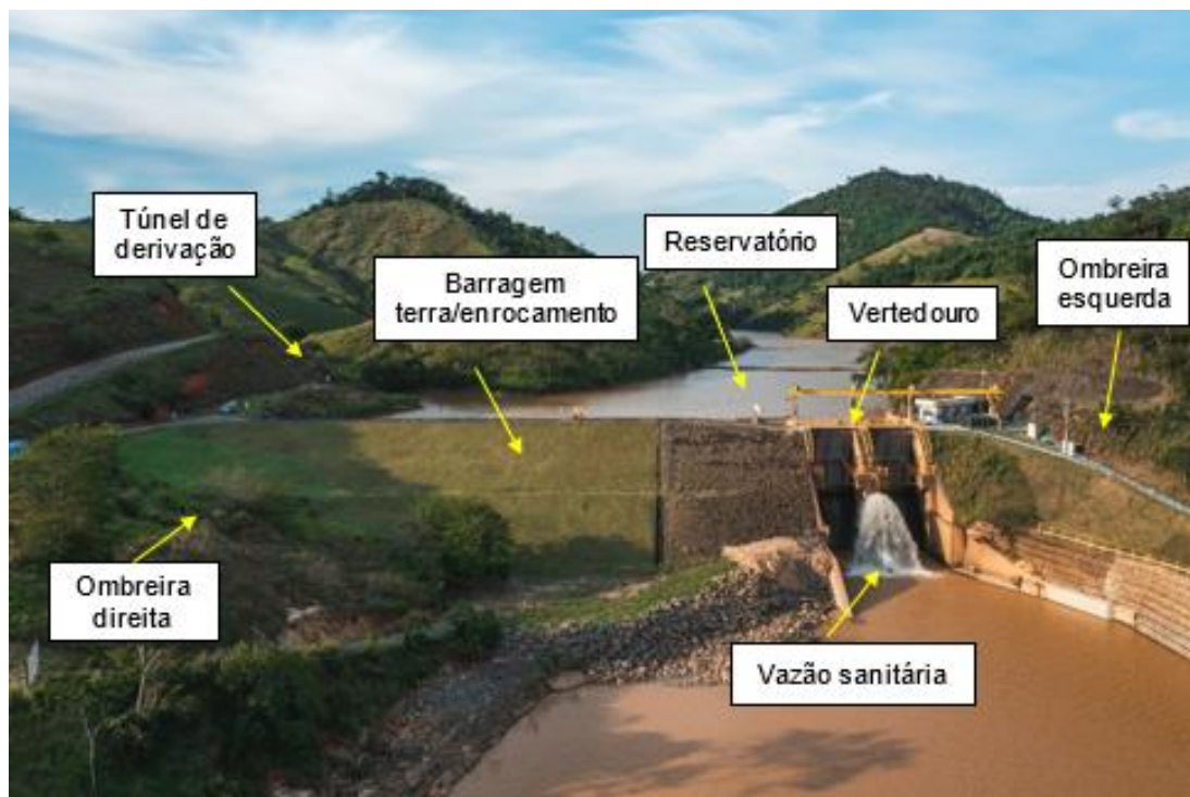
Imagem 1 – Arranjo geral da barragem de derivação
