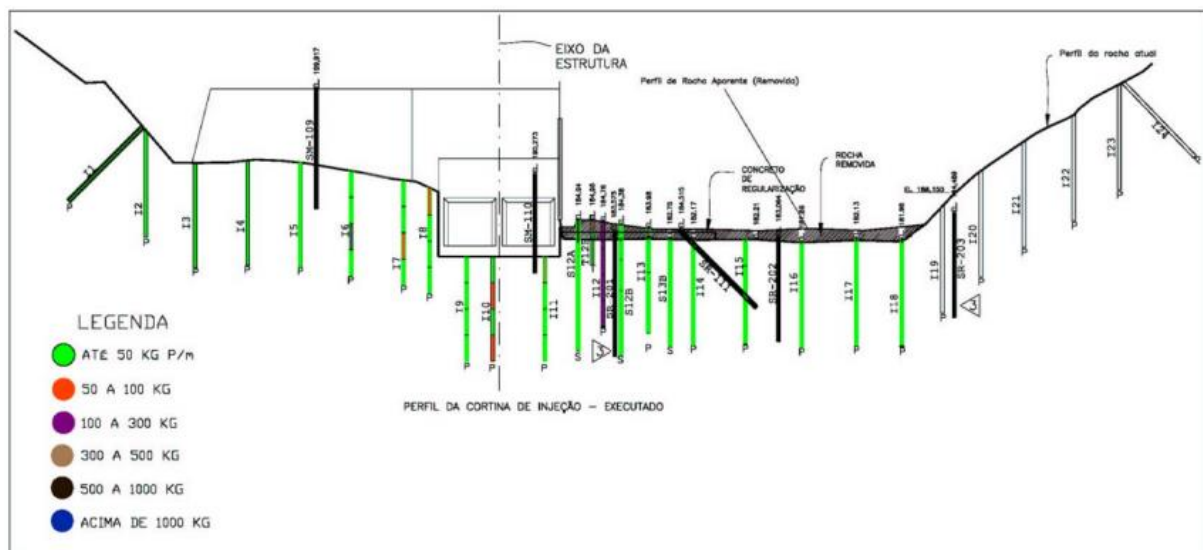
Figura 17 – Avaliação das condições da fundações
