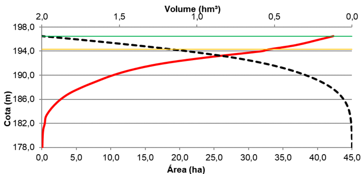
Figura 6 – Curva CAV do reservatório
