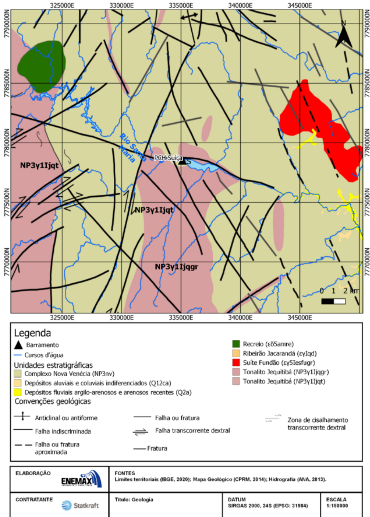
Figura 16 – Geologia regional
