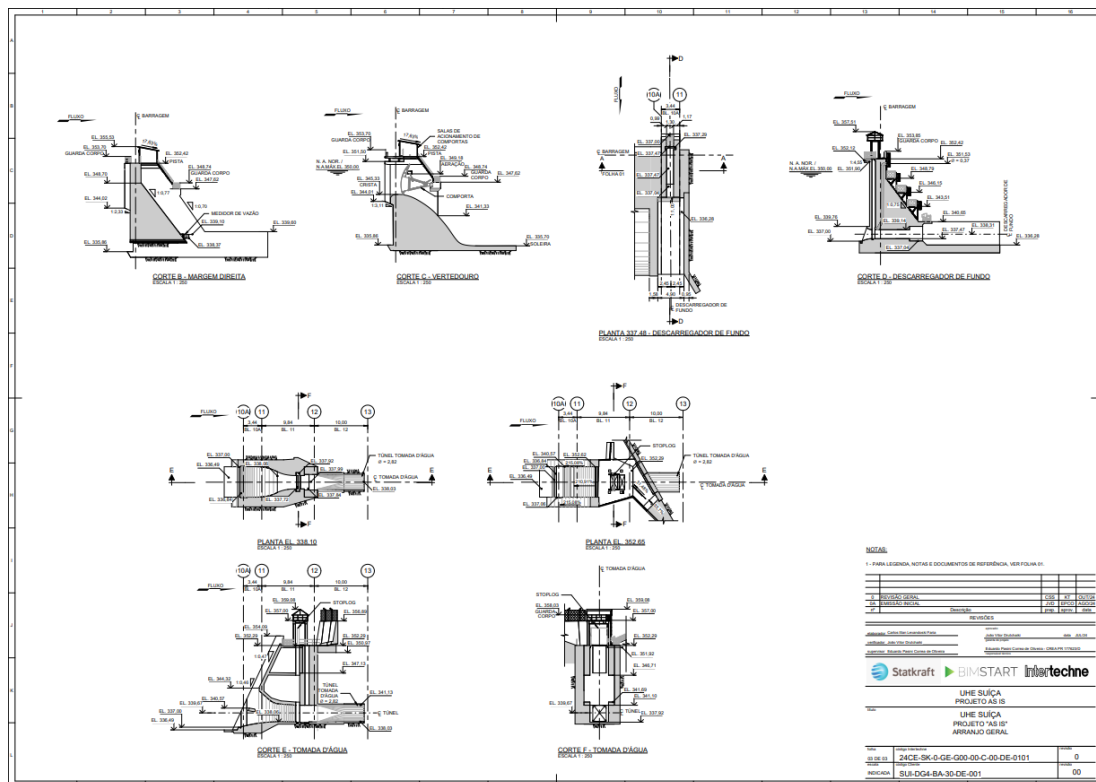
Figura 4 – Seções e detalhes da barragem – As Is
