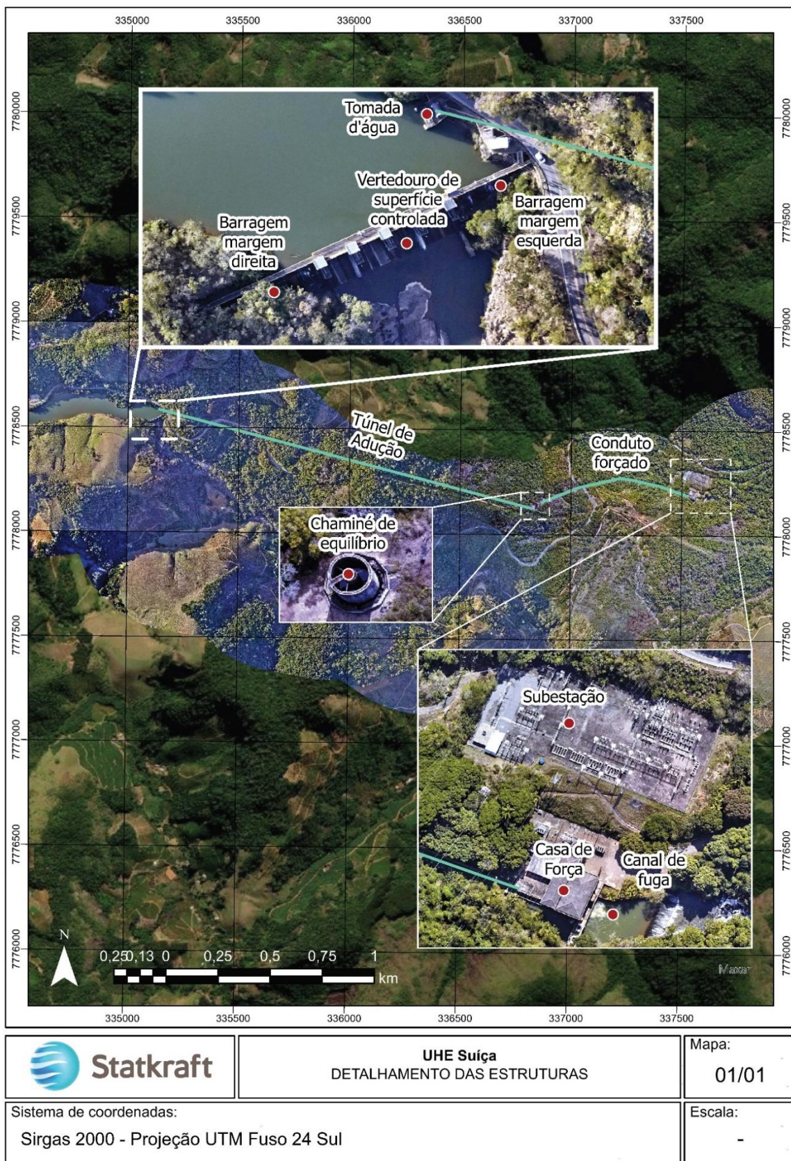
Figura 1 - Detalhamento das estruturas da UHE Suíça
