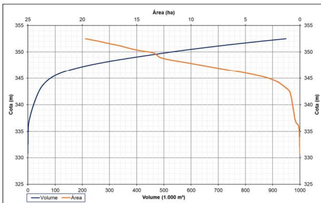
Figura 7 – Curva CAV do reservatório
