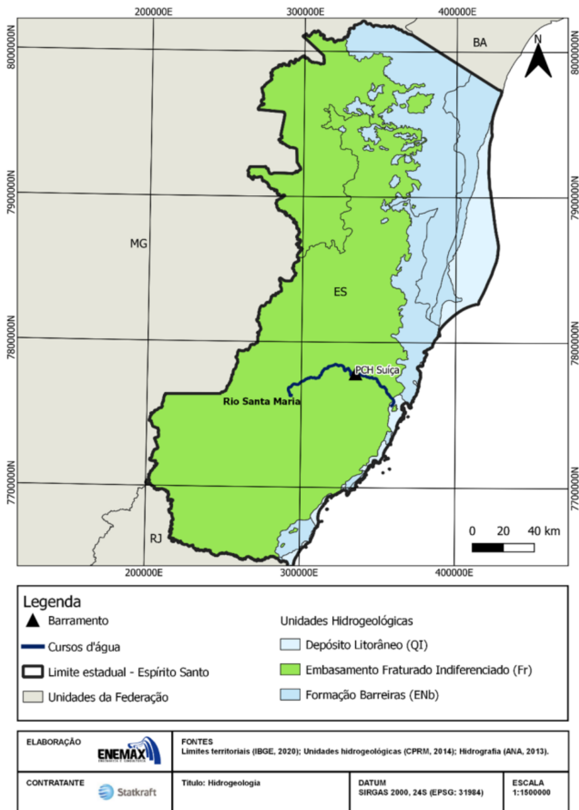
Figura 17 – Hidrogeologia
