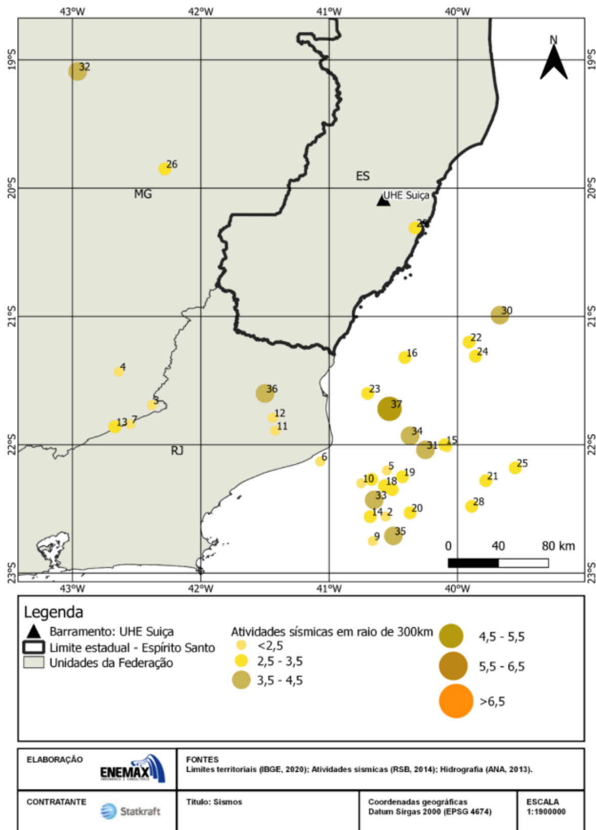
Figura 18 – Sismos
