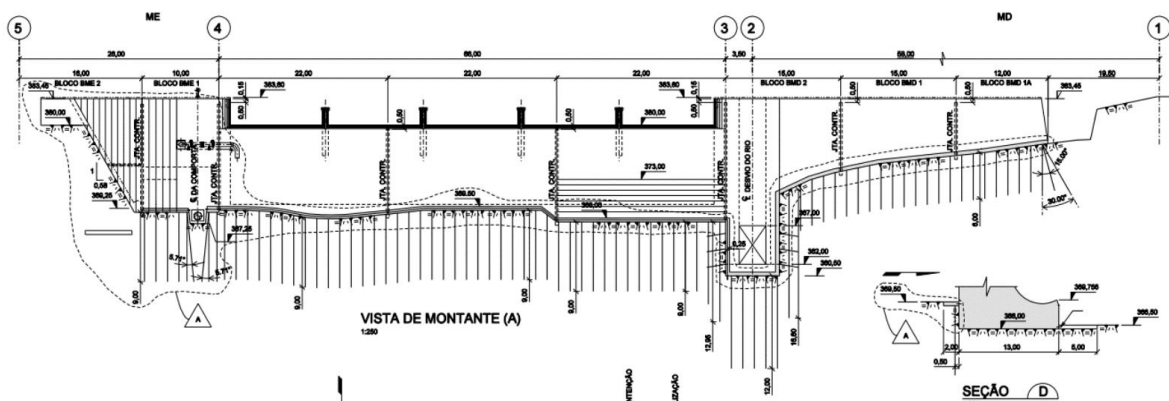
Figura 12 – Cortina de injeção na barragem
