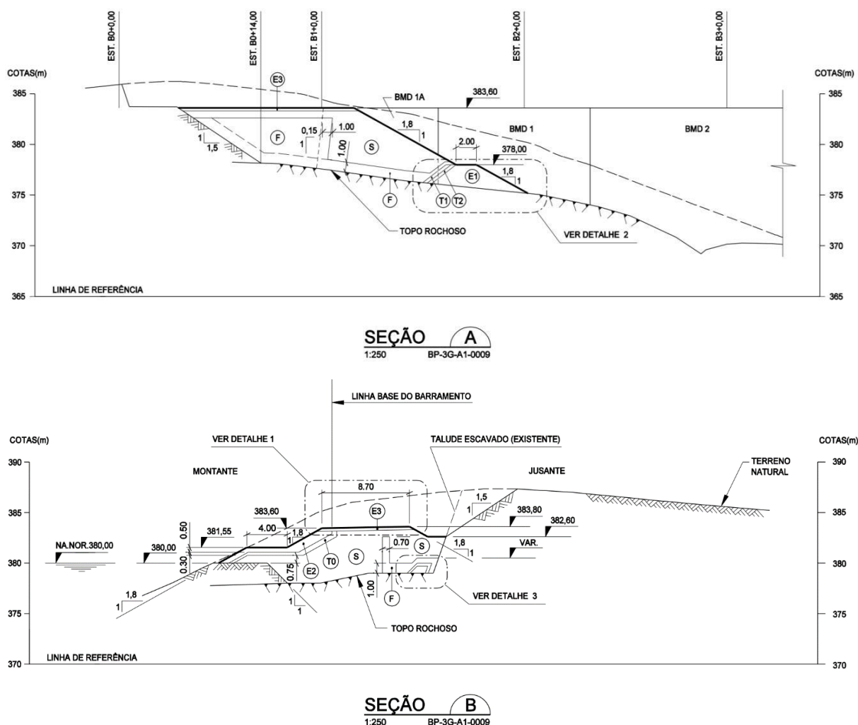
Figura 11 – Cortes da barragem de fechamento da margem direita
