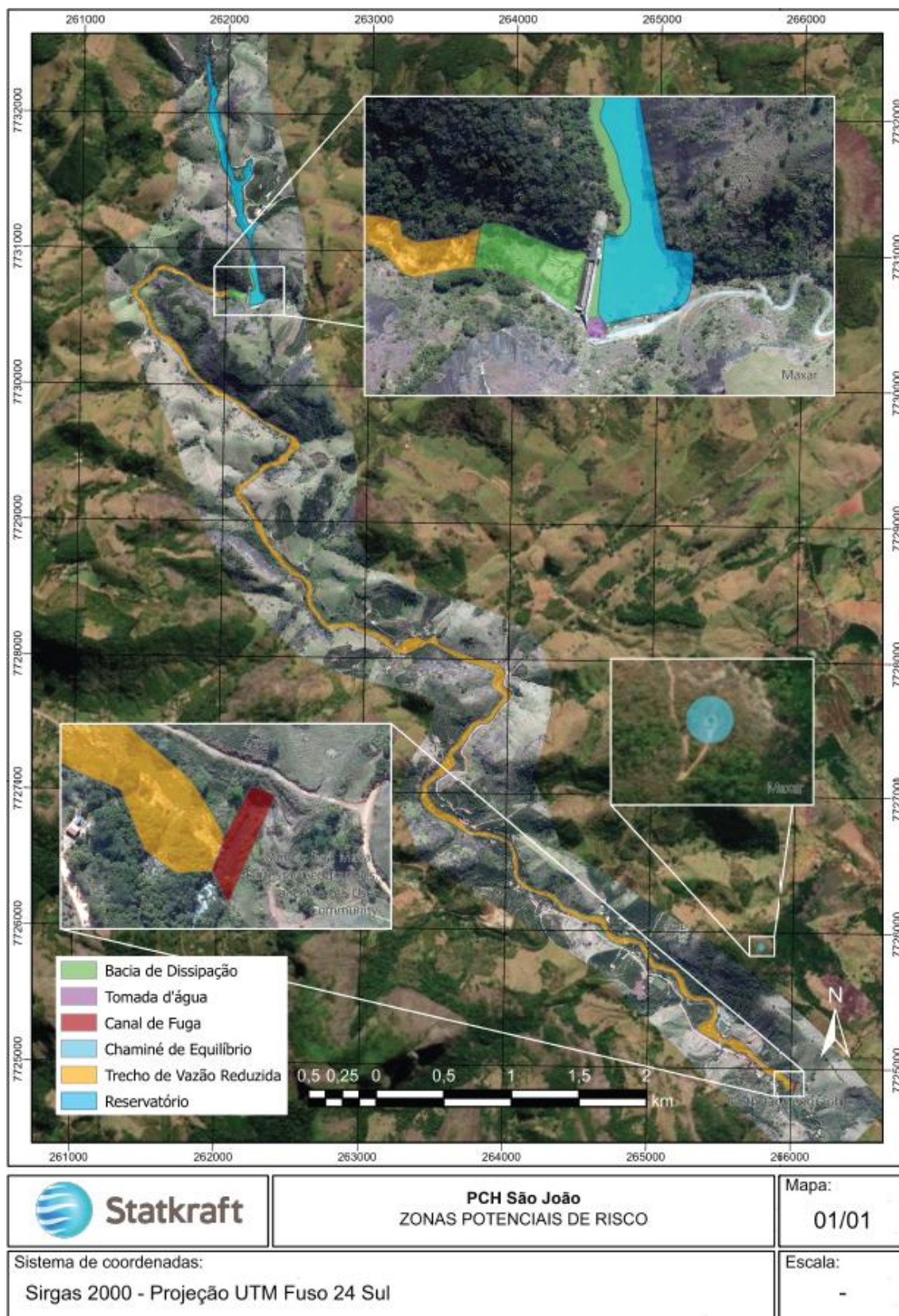
Figura 16 – Áreas de proteção junto as estruturas
