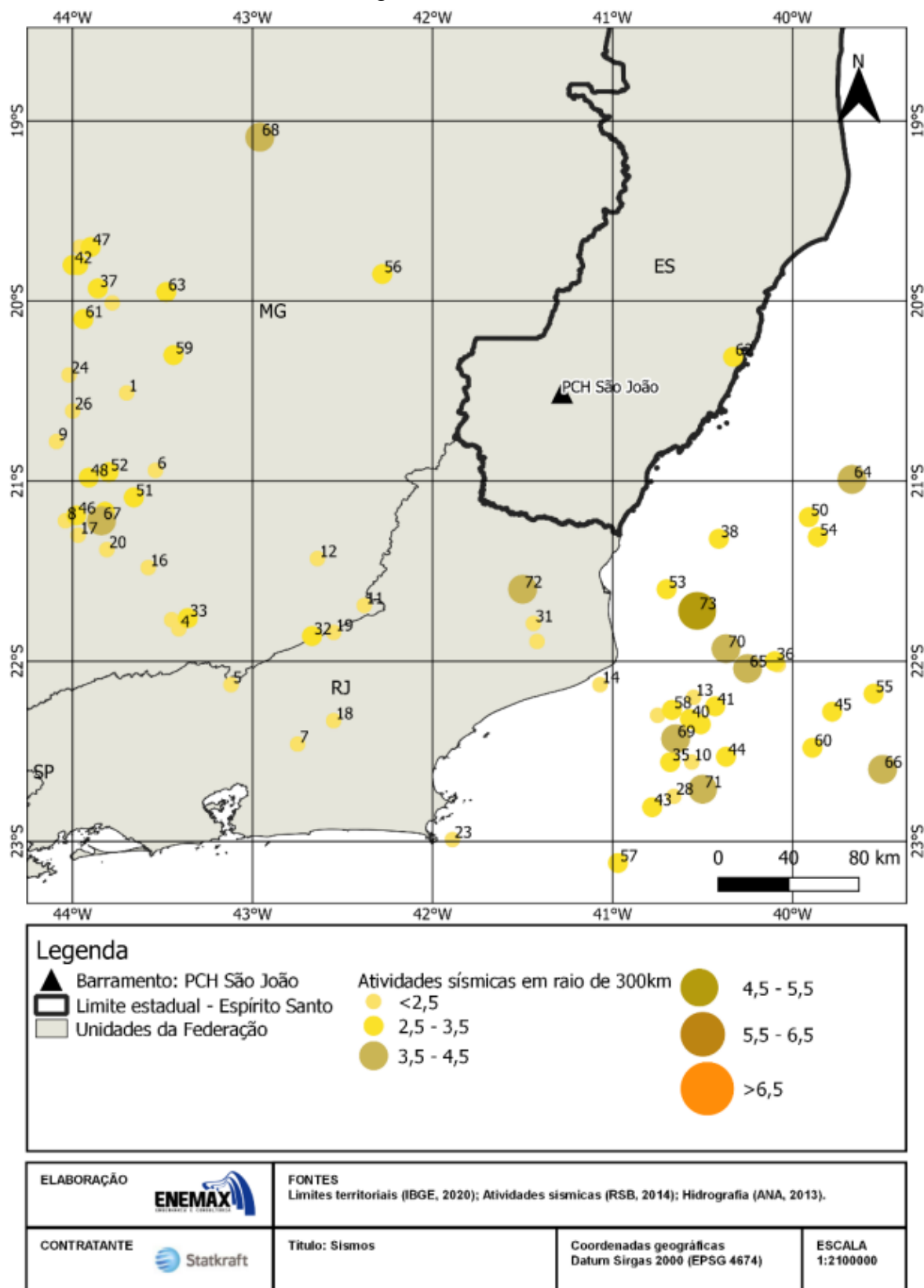
Figura 20 – Sismos
