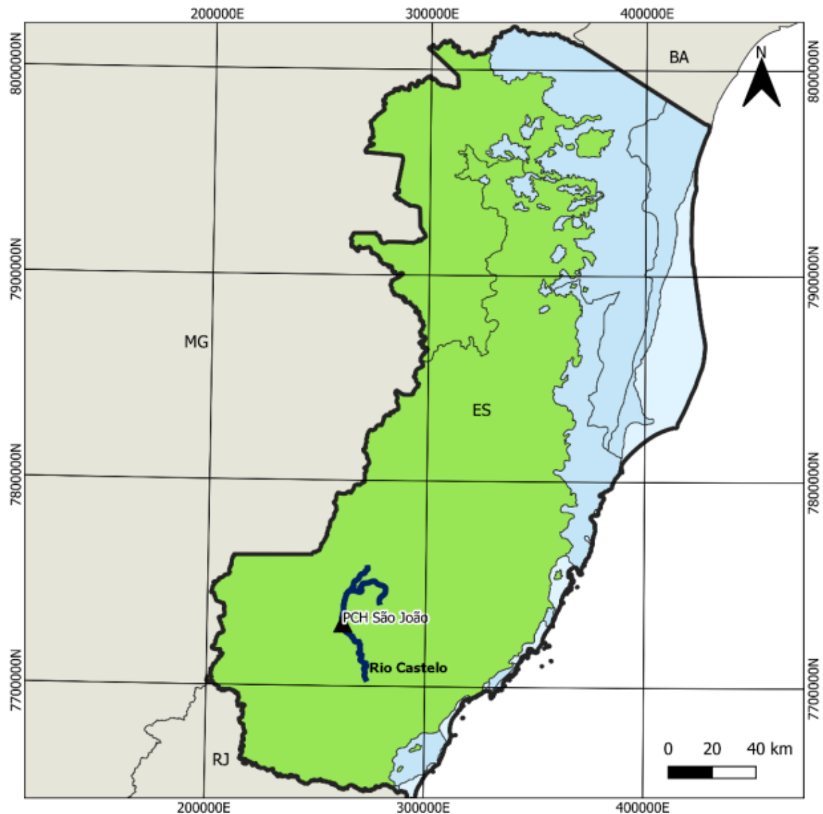
Figura 19 – Hidrogeologia
