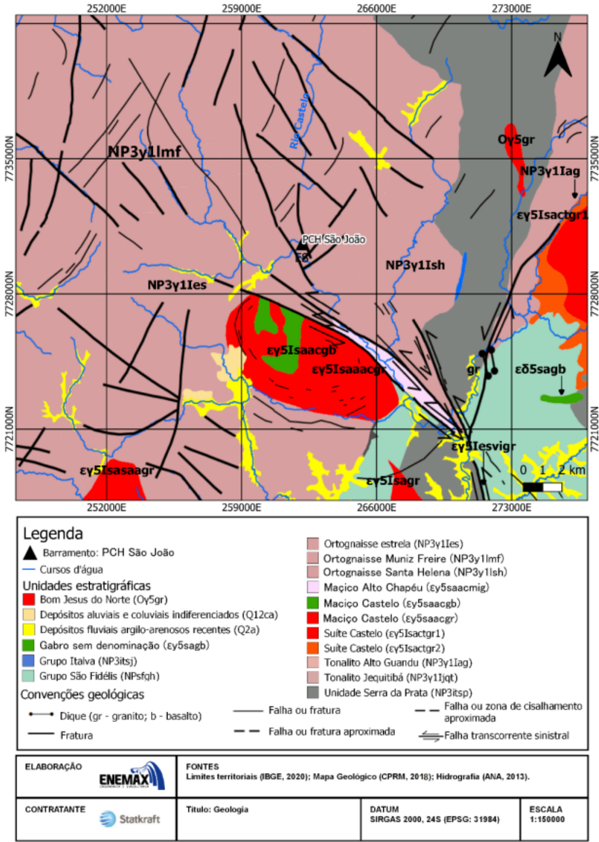
Figura 18 – Geologia regional
