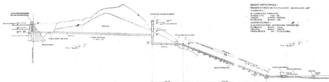
Figura 9 – Projeto executivo do sistema de adução
