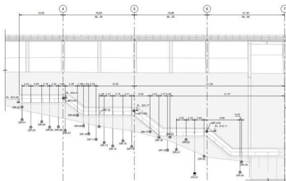
(a) Barragem da margem direita
