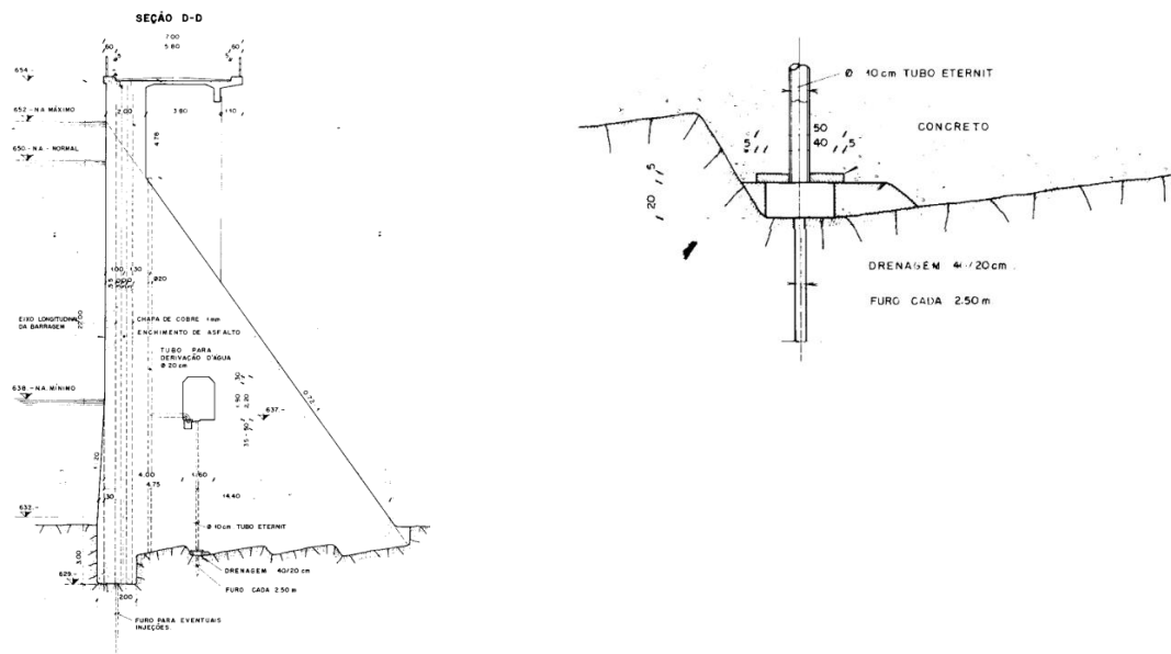
Figura 11 – Projeto executivo de tratamentos de fundação
