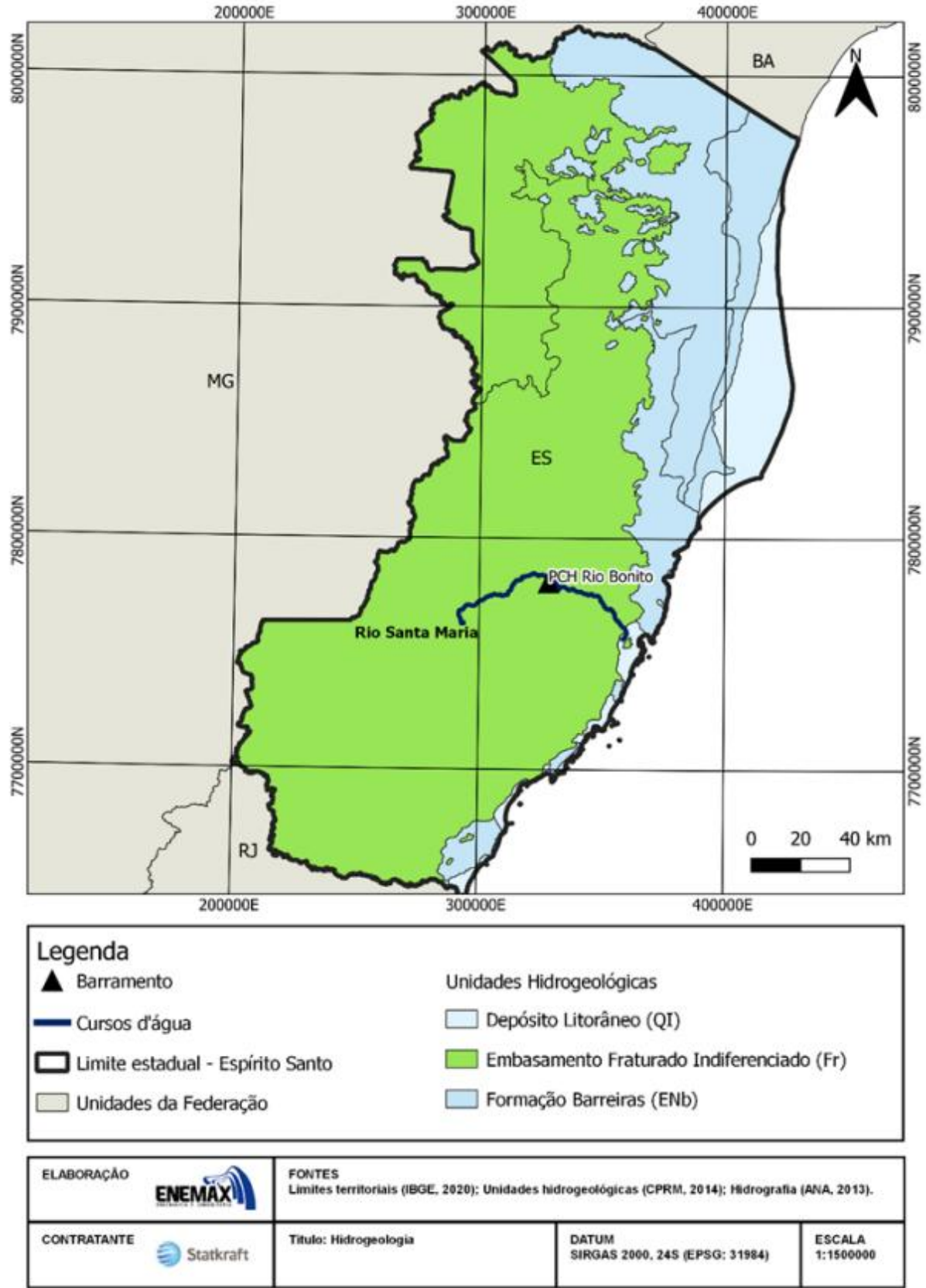
Figura 19 – Hidrogeologia
