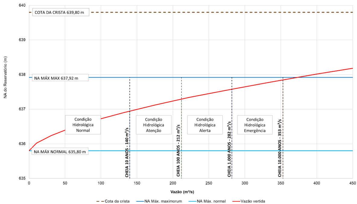
Figura 14 - Curva de Operação da barragem da PCH Rio Bonito
