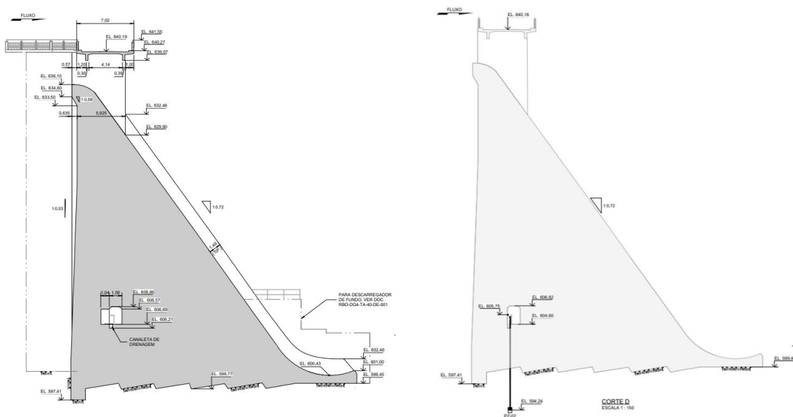
Figura 10 – Chavetas ao longo da fundação do vertedouro
