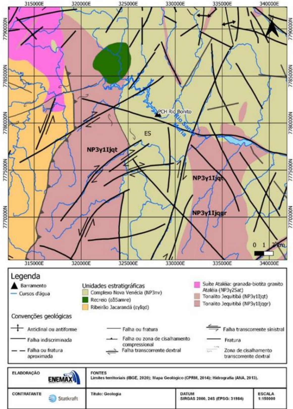
Figura 18 – Geologia regional
