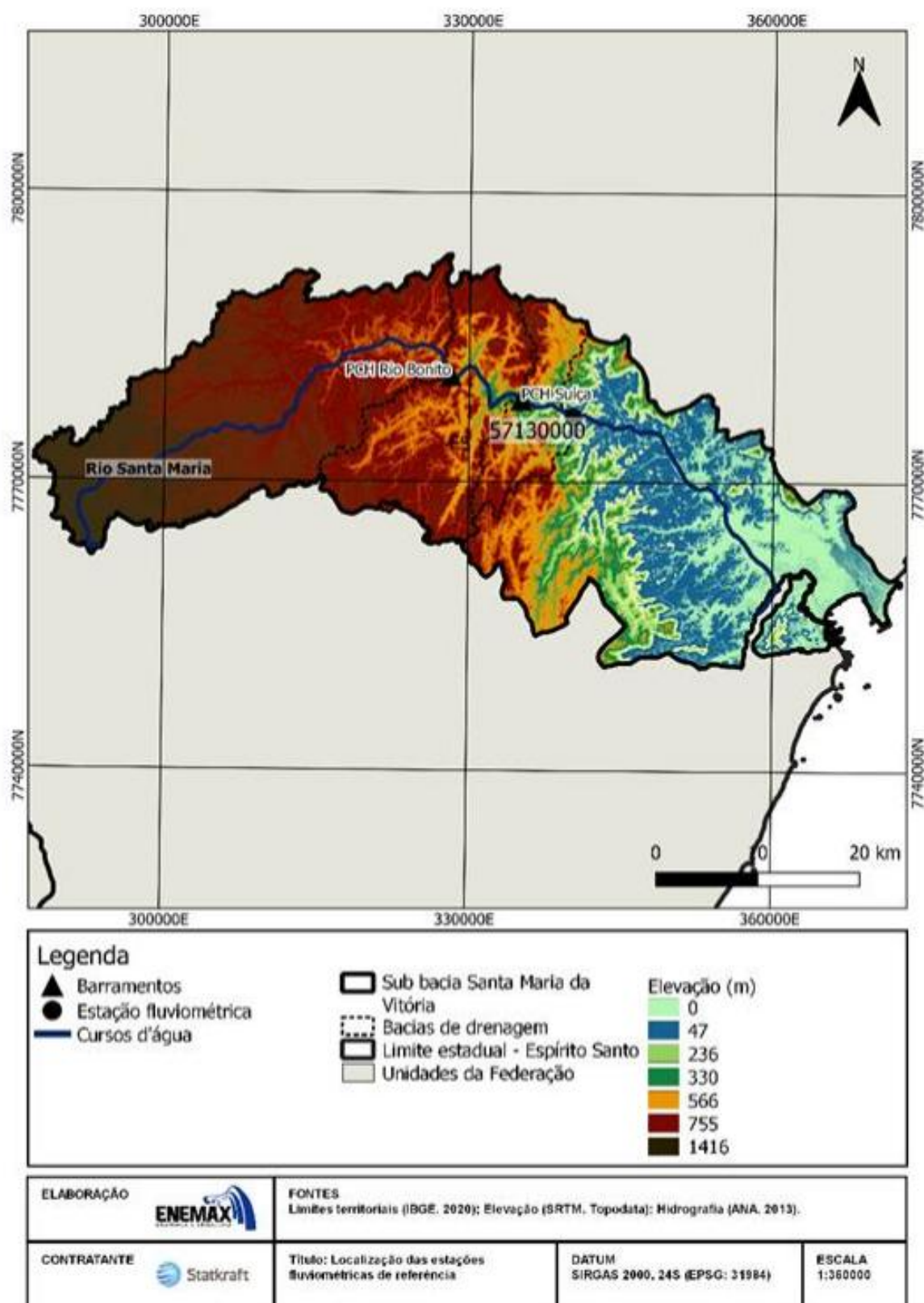
Figura 17 – Bacia hidrográfica do rio Santa Maria da Vitória
