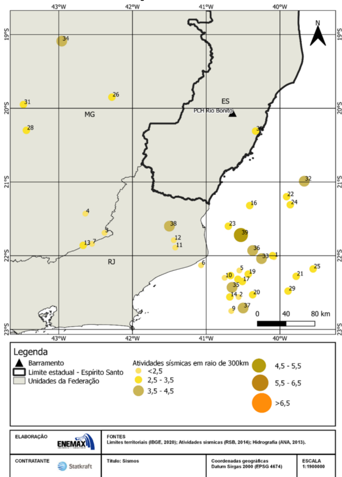
Figura 20 – Sismos
