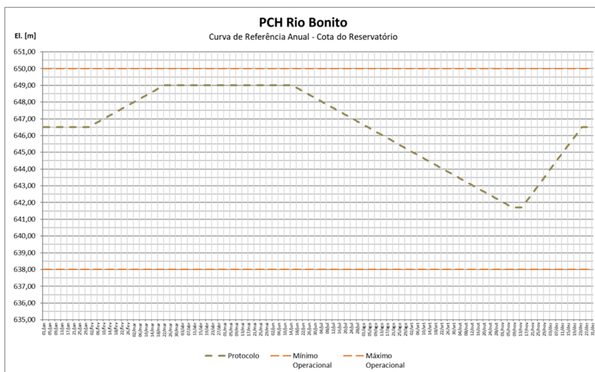
Figura 15 - Curva de referência anual
