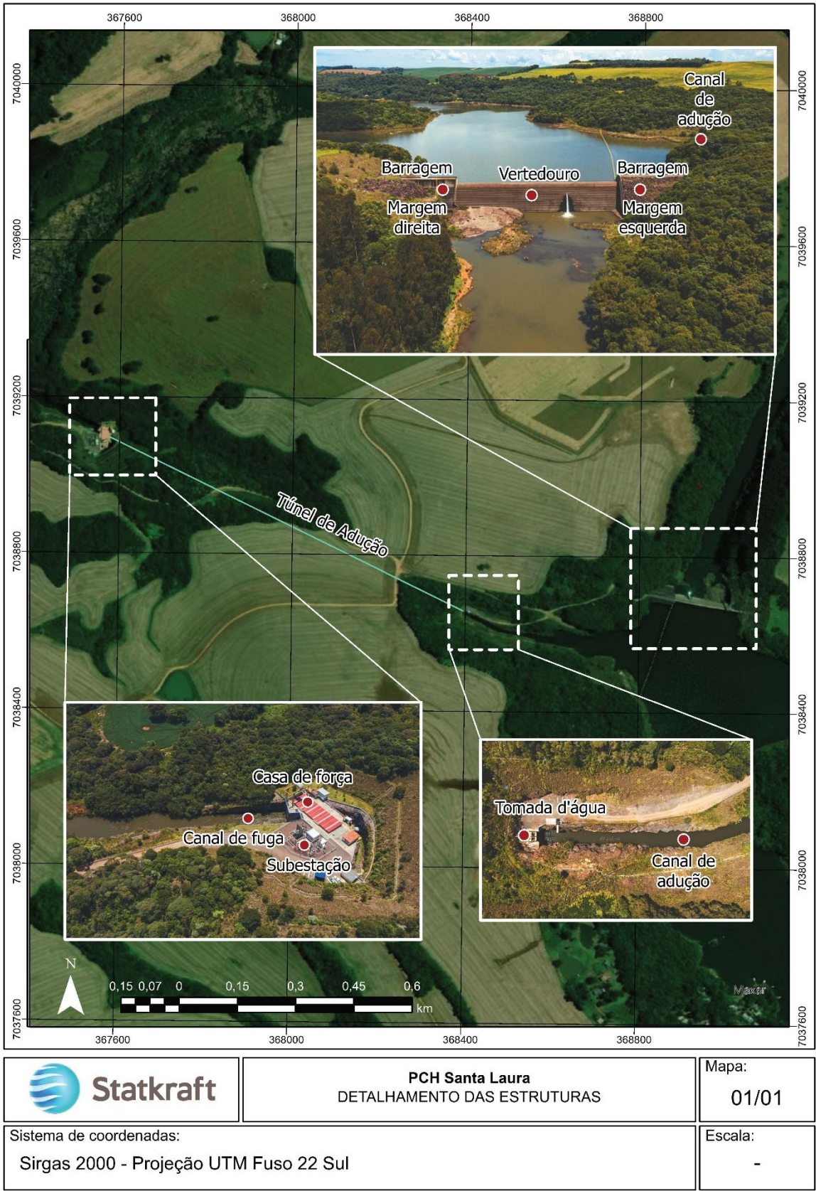
Figura 1 - Detalhamento das estruturas da PCH Santa Laura
