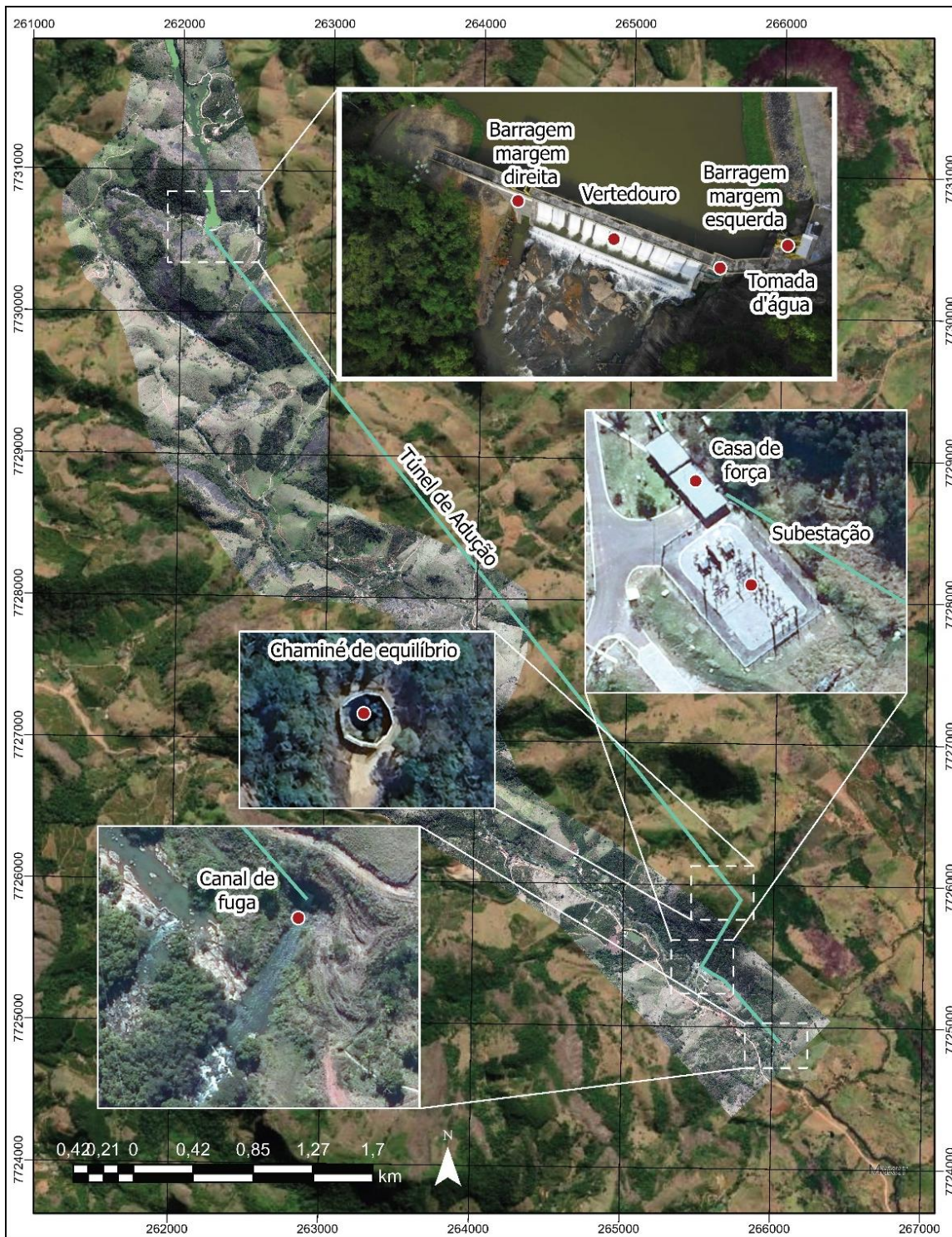
Figura 1 - Detalhamento das estruturas da PCH São João
