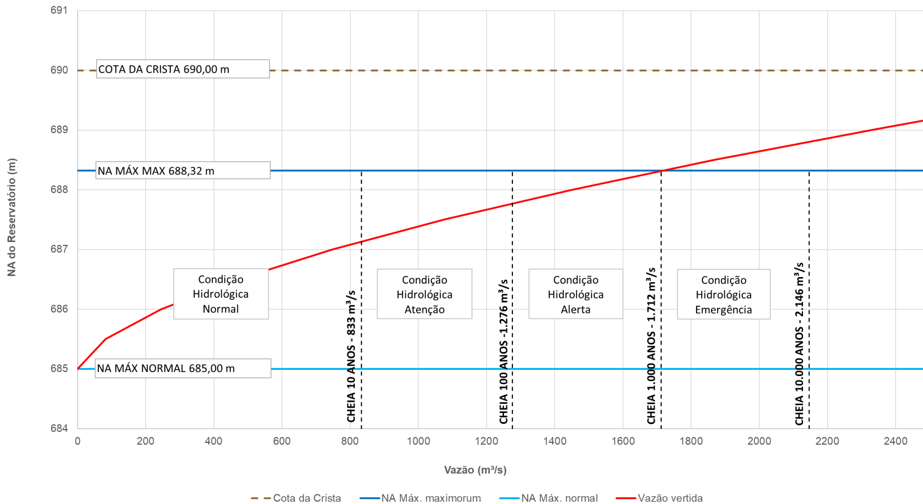
Figura 3 - Curva de Operação da barragem da PCH Santa Laura
