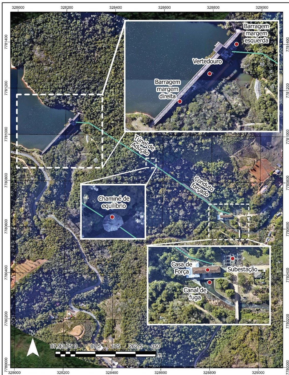
Figura 1 - Detalhamento das estruturas da PCH Rio Bonito
